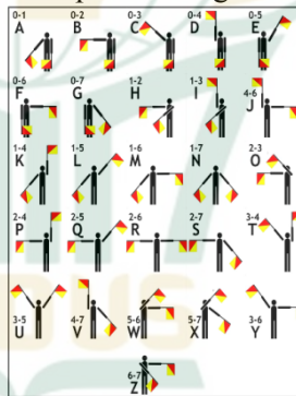
Gambar 4.12 Rumus Semaphore 98
