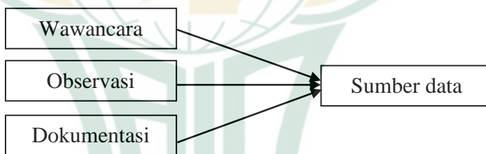
Gambar 3.2 Triangulasi Sumber
