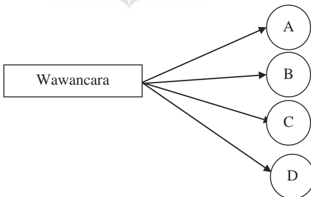
Gambar 3.2 Triangulasi Sumber
