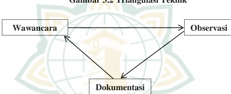
Gambar 3.2 Triangulasi Teknik
