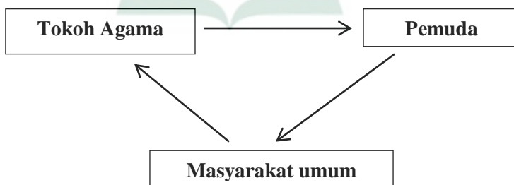
Gambar 3.1 Triangulasi Sumber
