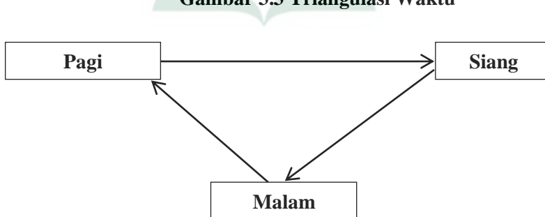
Gambar 3.3 Triangulasi Waktu
